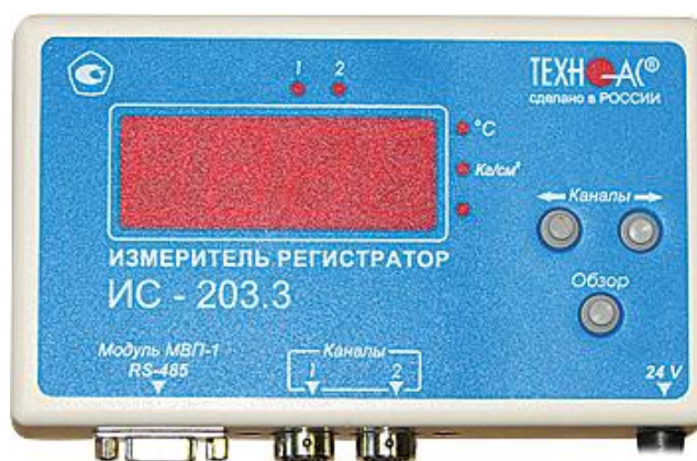
Рисунок 3 - Фотография общего вида прибора ИС-203.3
