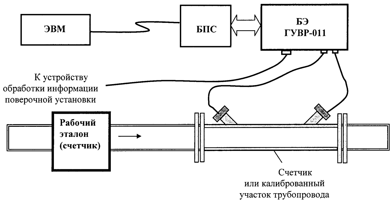
Рисунок Б.2 — Поверочная установка с эталонными счетчиками газа
