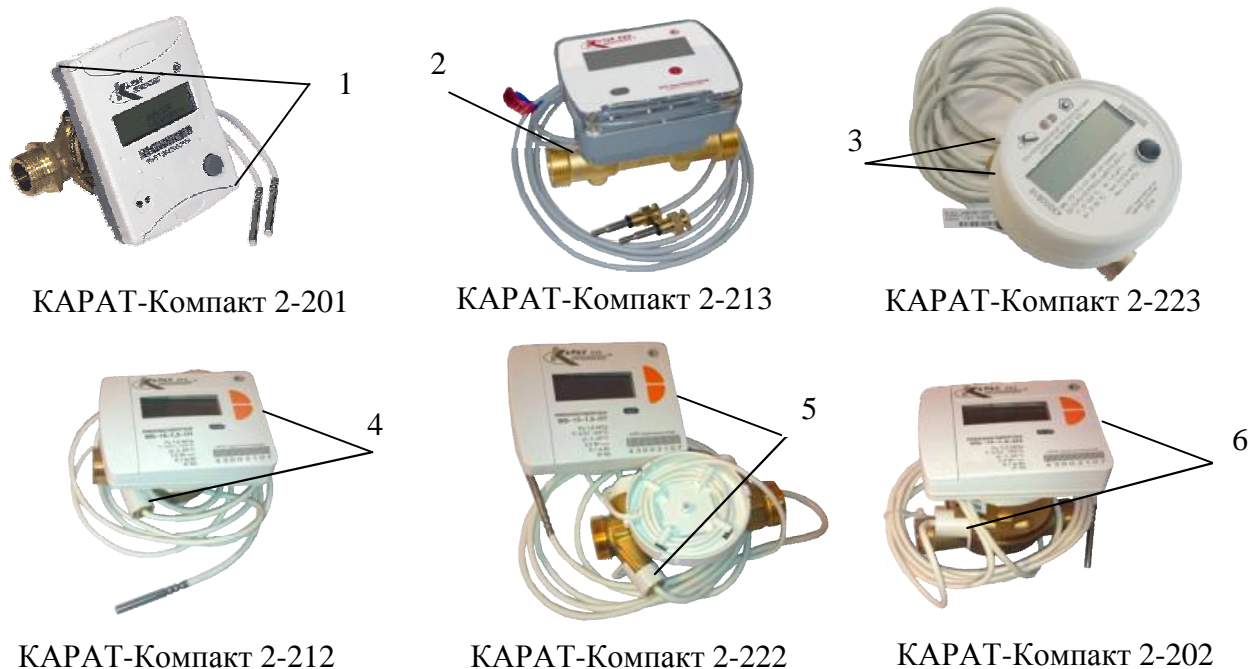
1 – 6 Места пломбирования при выпуске из производства Рисунок 1 – Внешний вид теплосчетчиков KARAT-Компакт 2 и места их пломбирования
