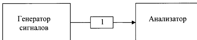
1 – фильтр (для подавления 2f_1 )
