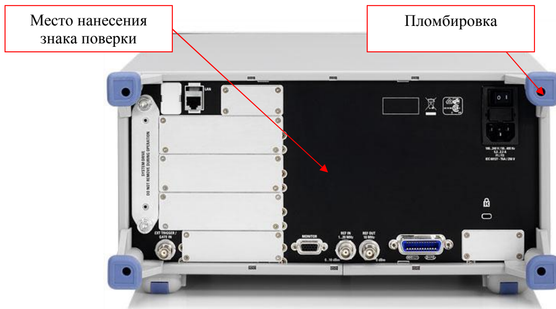
Рис. 2 - Схема пломбировки от несанкционированного доступа и нанесения знака поверки.
