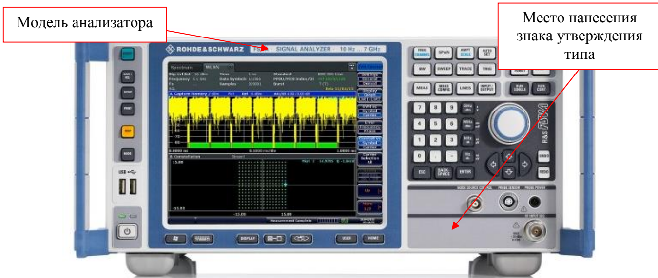
Рис. 1 - Внешний вид анализаторов спектра FSVA4, FSVA7, FSVA13, FSVA30, FSVA40
