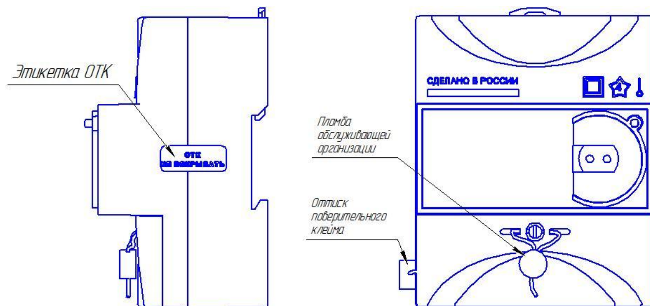
Рисунок 2 – Схема пломбирования и место нанесения знака поверки на счетчики.
