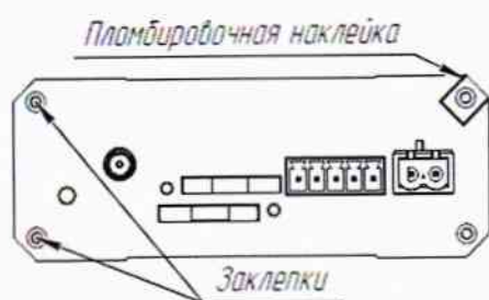
а) вид спереди
