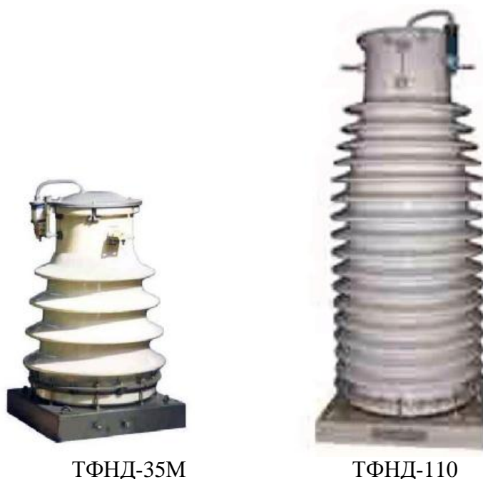
Рисунок 1 - Фотографии общего вида трансформаторов тока ТФНД.
