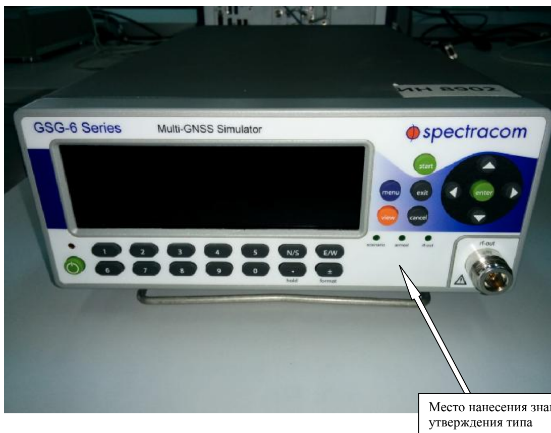
Рисунок 1 - Внешний вид имитатора (передняя панель)
