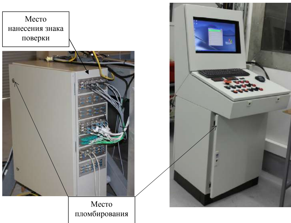
Рисунок 1 - Внешний вид ПТК и автоматизированного рабочего места оператора с указанием мест пломбировки и нанесения знака поверки
