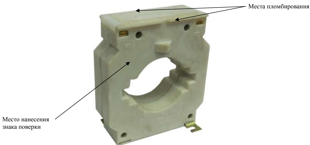
Рисунок 1 – Внешний вид трансформаторов тока ТШП-СЭЦ-0,66
