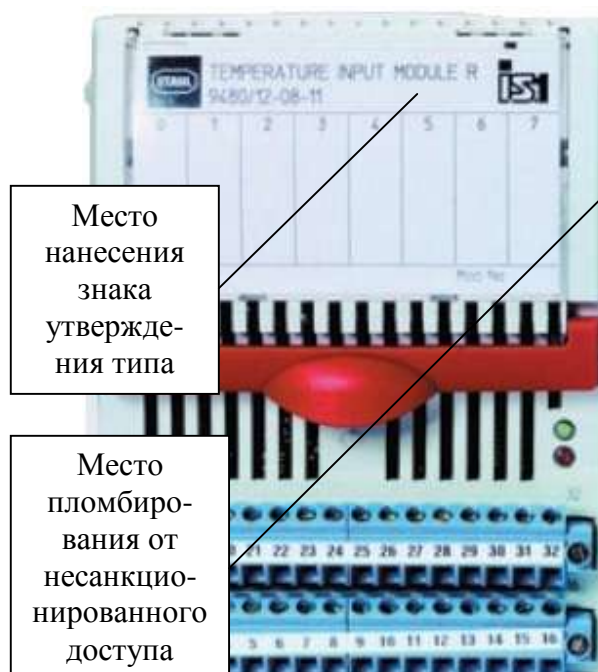
Рисунок 2 – Модули 9480
