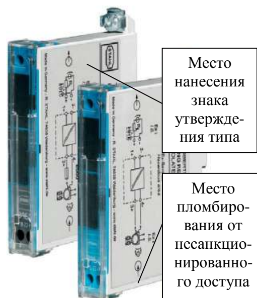
Рисунок 6 – Модули 9164
