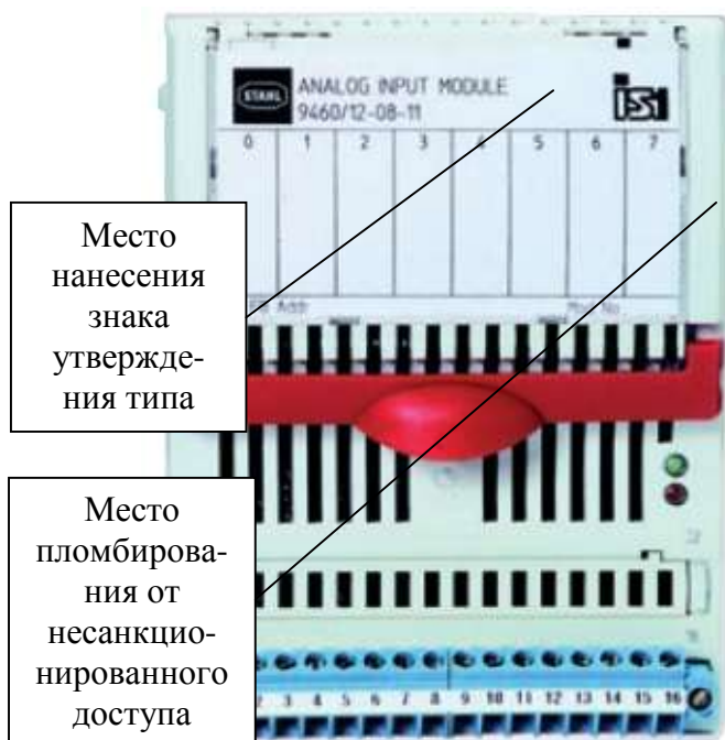
Рисунок 1 – Модули 9460, 9461, 9465, 9466, 9481
