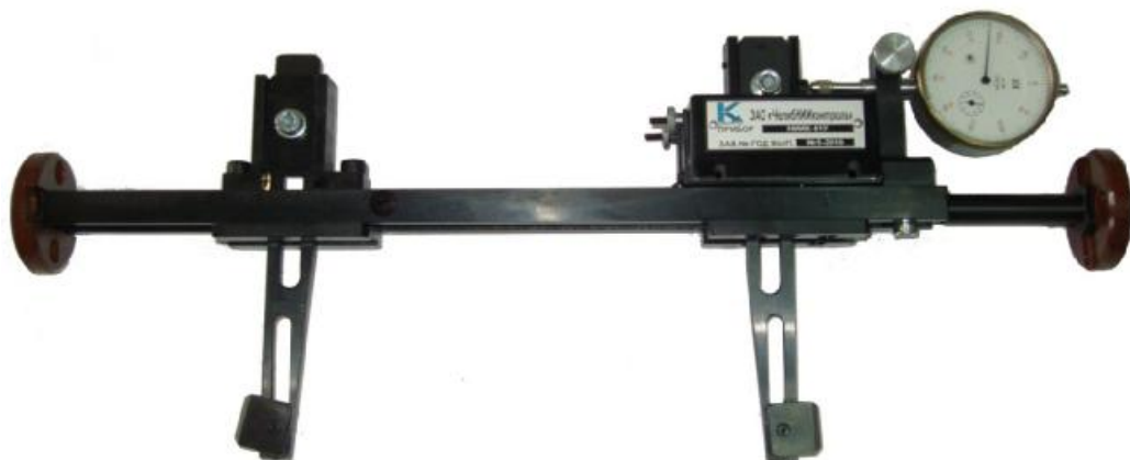
Рисунок 8 – Общий вид прибора исполнения НИИК-100/01У-01
