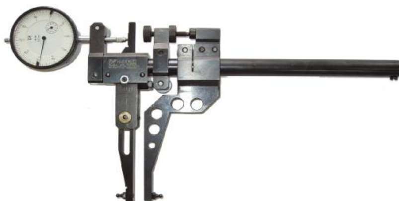
Рисунок 10 – Общий вид прибора НИИК-100/32
