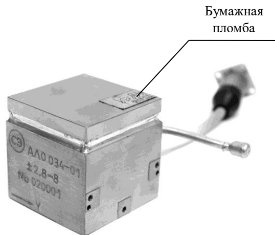
Рисунок 1 – Общий вид акселерометра
