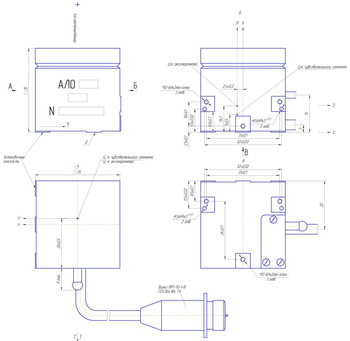
Рисунок 2 – Габаритно-установочные размеры акселерометра
