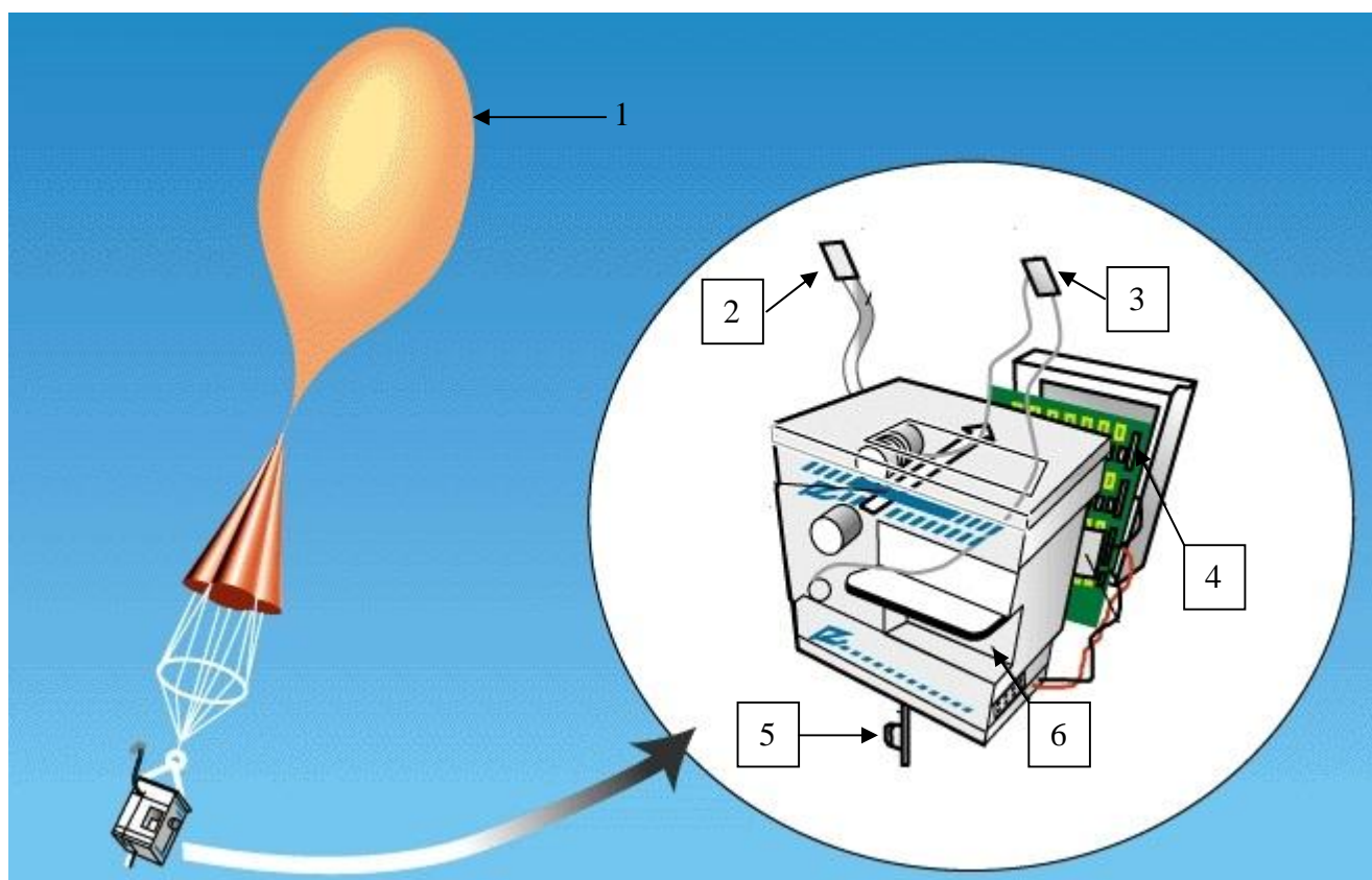
Рисунок 1 - Общий вид радиозондов цифровых аэрологических ЦРЗ-МРК 1 – оболочка, 2 - термометр сопротивления (терморезистор), 3 – емкостной преобразователь относительной влажности, 4 – радиоблок, 5 - антенна, 6 – аккумуляторная батарея
