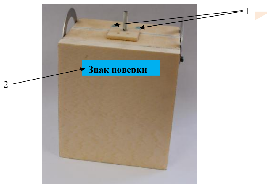
Рисунок 2 - Схема пломбирования радиозондов цифровых аэрологических ЦРЗ-МРК и место нанесения знака поверки 1 – пломбы на корпусе радиозонда 2 – место нанесения знака поверки.
