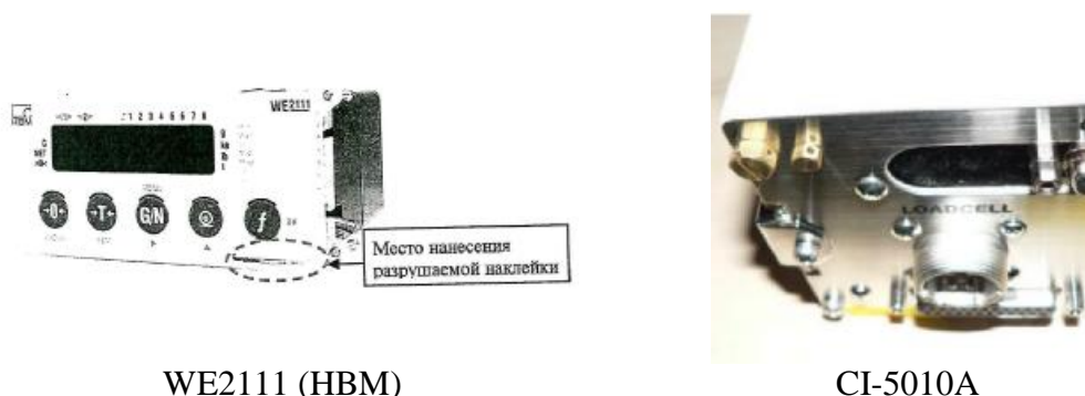
Рисунок 5 - Схема пломбировки приборов весоизмерительных
