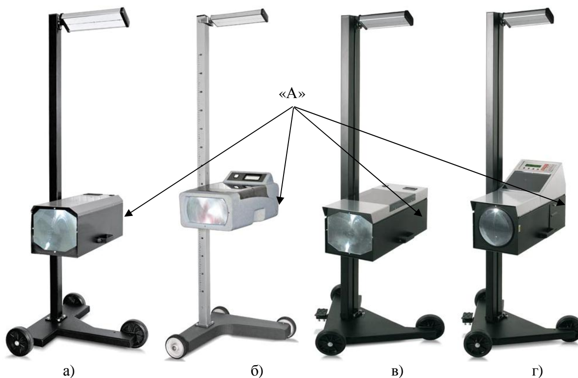
Рисунок 1 - Общий вид приборов для измерений параметров света фар автотранспортных средств TECO HL185 (а), TECO HL190 PLUS (б), TECO HL200 (в), TECO HL225 (г)
