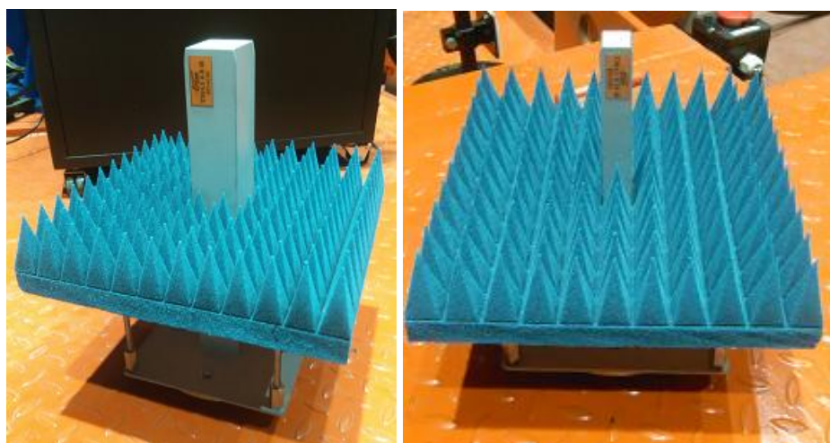
Рисунок 6 – Внешний вид антенн-зондов диапазона частот от 4 до 18 ГГц
