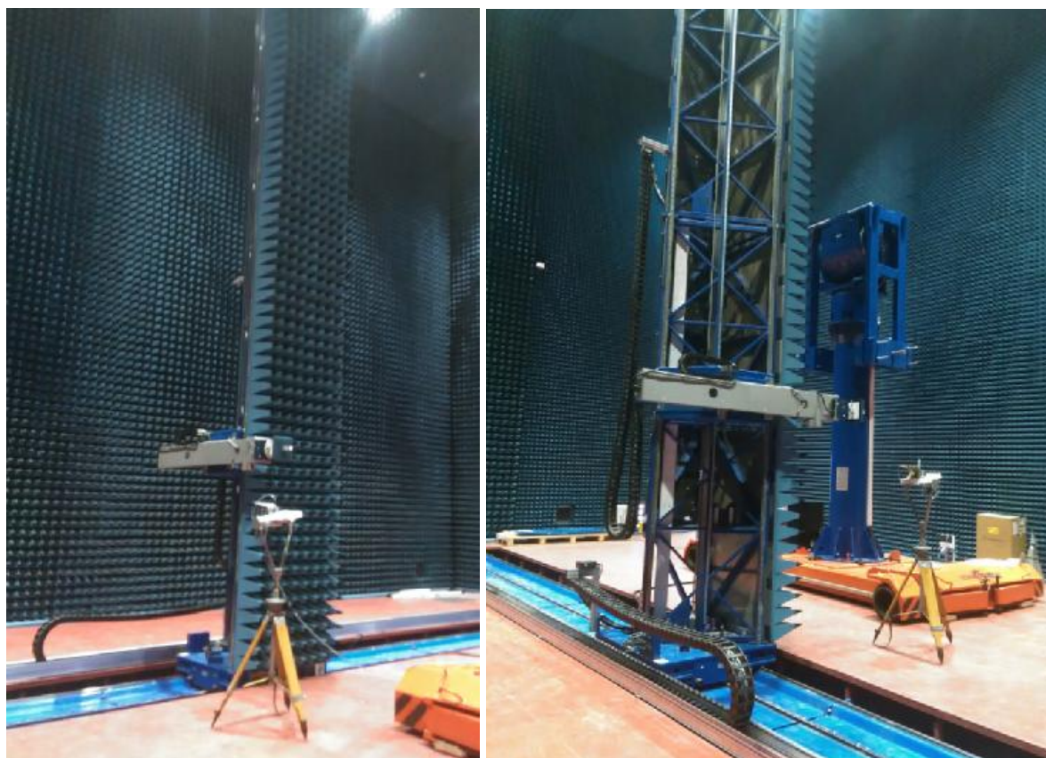
Рисунок 1 – Внешний вид сканера с установленной антенной-зондом
