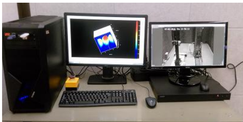
Рисунок 7 – Внешний вид рабочего места оператора с ПЭВМ, предназначенной для управления работой комплекса и обработки результатов измерений
