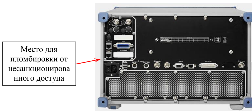
Рисунок 8 – Задняя панель векторного анализатора цепей
