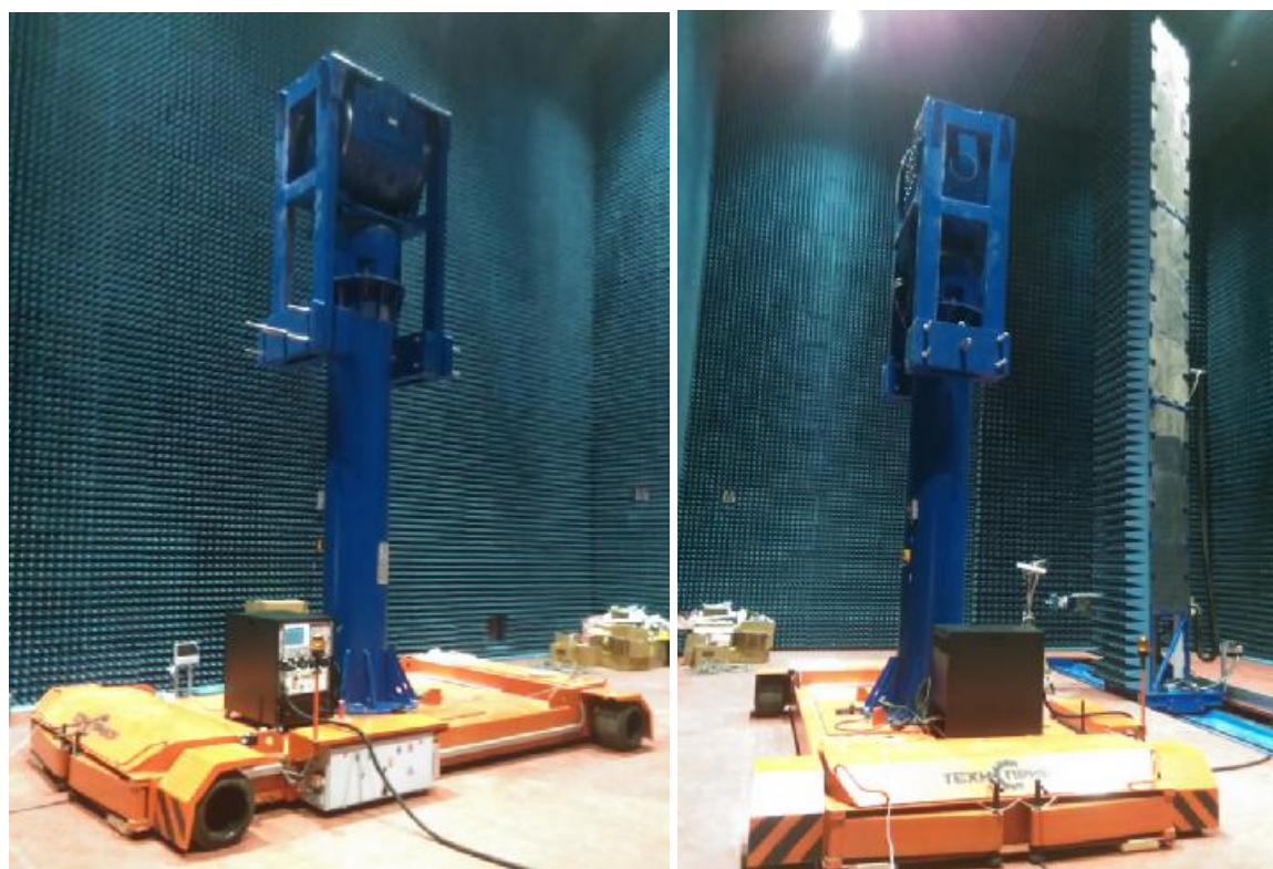
Рисунок 2 – Внешний вид ОПУ и сканера
