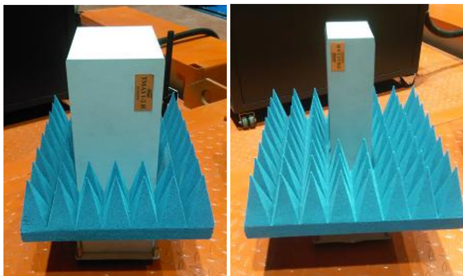
Рисунок 5 – Внешний вид антенн-зондов диапазона частот от 1 до 4 ГГц
