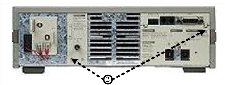
Примечание: ② - места пломбировки от несанкционированного доступа. Рисунок 7 – Источник питания (модель 6672А). Вид сзади
