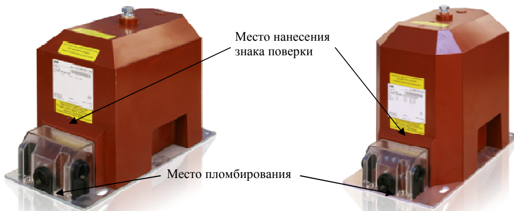
Рисунок 1 – Внешний вид трансформаторов напряжения ТЭС 4 и ТЭС 5
