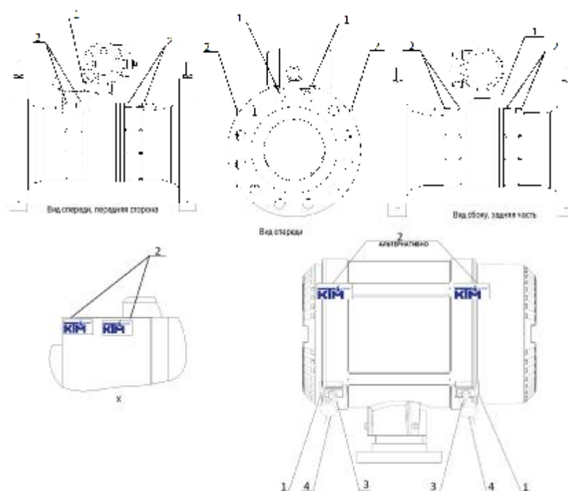
Рисунок 2 – Схема пломбирования (места нанесения знака поверки);
