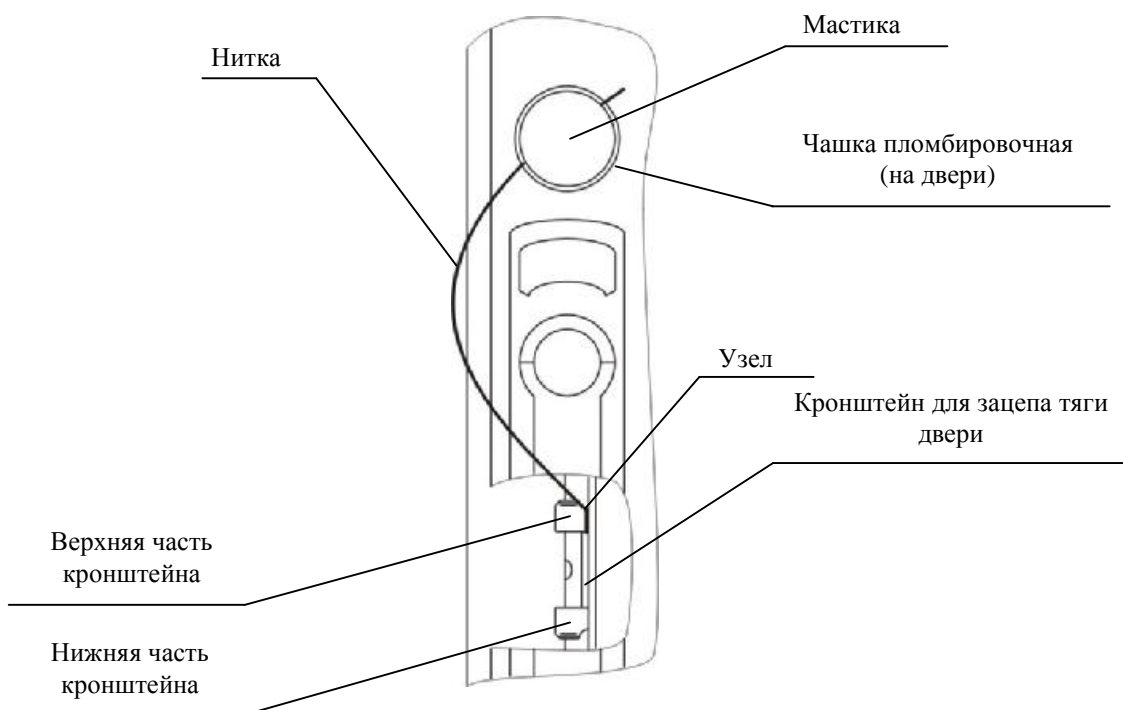
Рисунок 2 – Схема защиты от несанкционированного доступа
