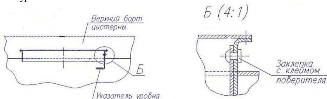
Рисунок 2 - Обозначение места для нанесения оттиска поверительного клейма
