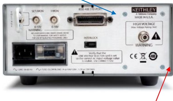
Рисунок 3 – Задняя панель модели 2290E-5
