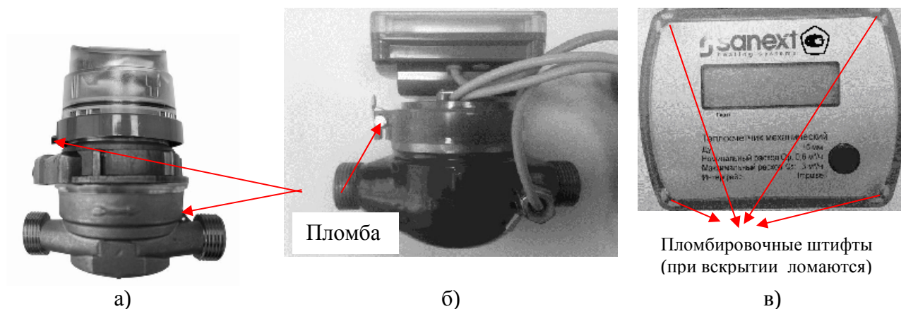
Рисунок 1 - Теплосчётчики Sanext серии М
