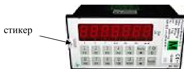
Рисунок 8 – Вид терминала MC 302 с указанием места пломбировки
