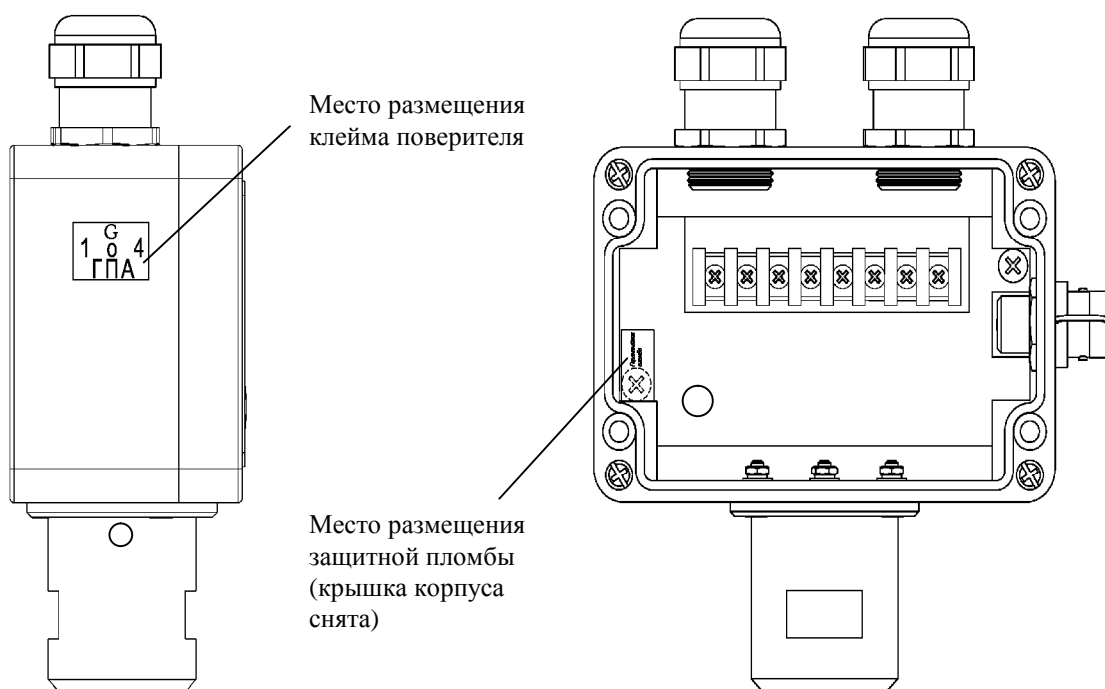
Рисунок 2 – Схема пломбировки сигнализаторов от несанкционированного доступа и размещения оттиска клея поверителя
