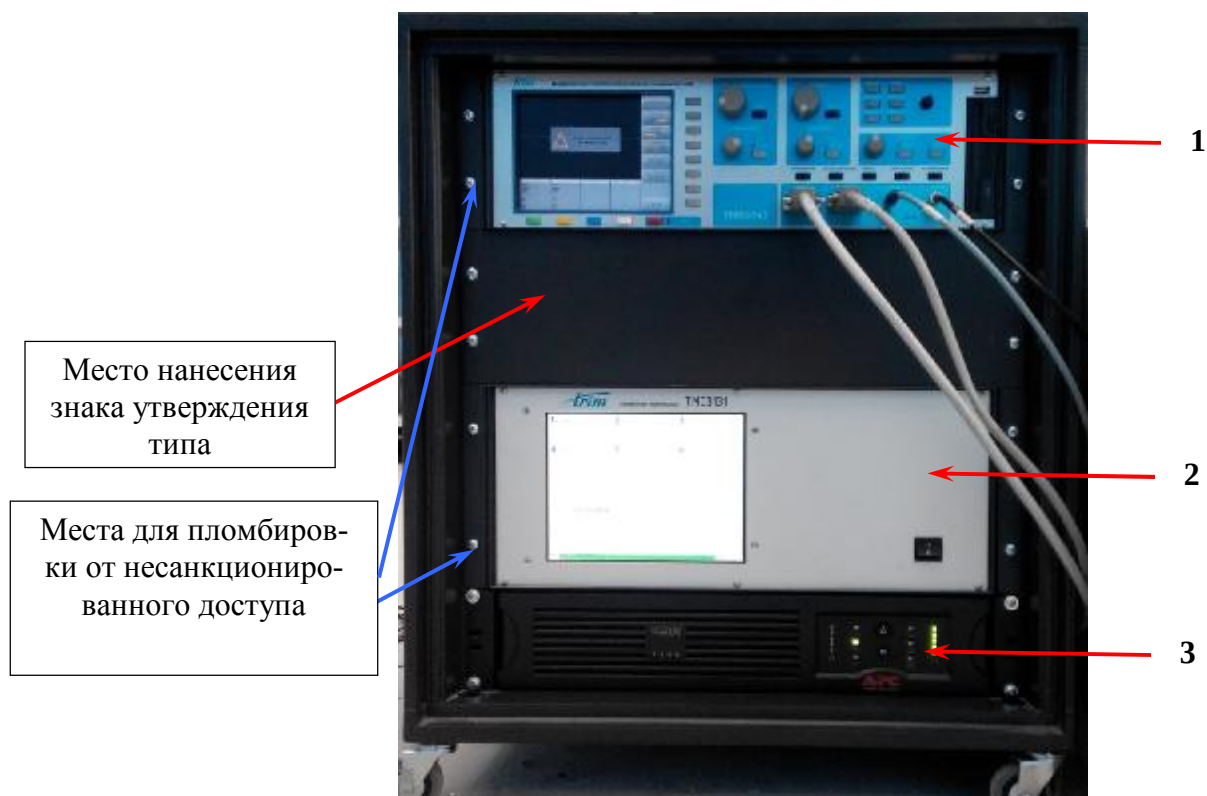
Рисунок 2 – Схематичный вид ОПУ
