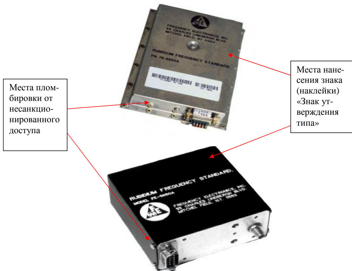
Рисунок 1 – Внешний вид стандартов FE-5650A, FE-5680A
