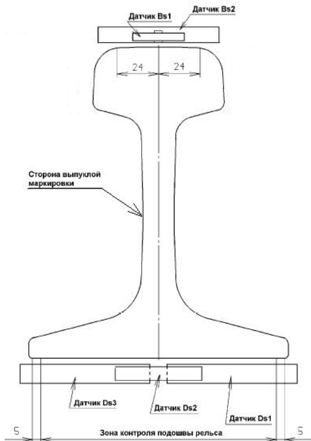
Рисунок 3 – Статические ВТП
