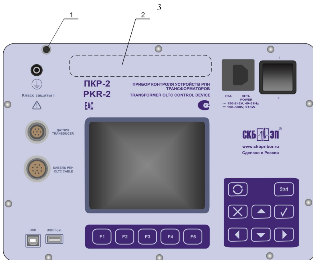
Рис. 3 Схема панели
