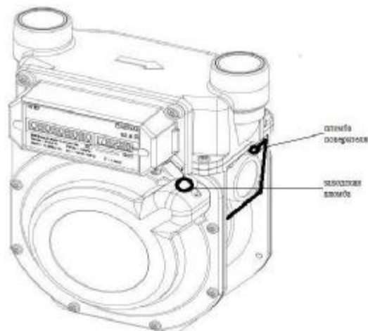
Рисунок 1. Схема пломбировки счетчика газа
