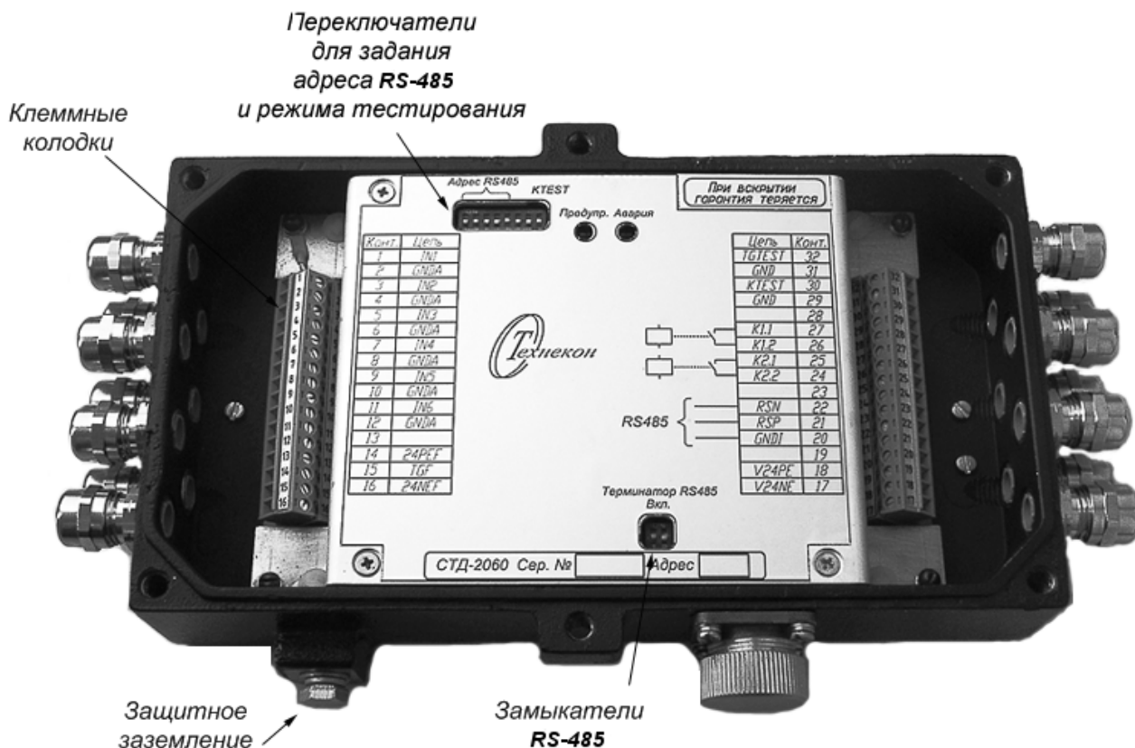
Рисунок 5 - Внешний вид контрольно-измерительного блока STD-2060 со снятой верхней крышкой
