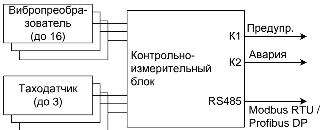
Рисунок 1 – Структурная схема измерителя вибрации многоканального СТД-2060
