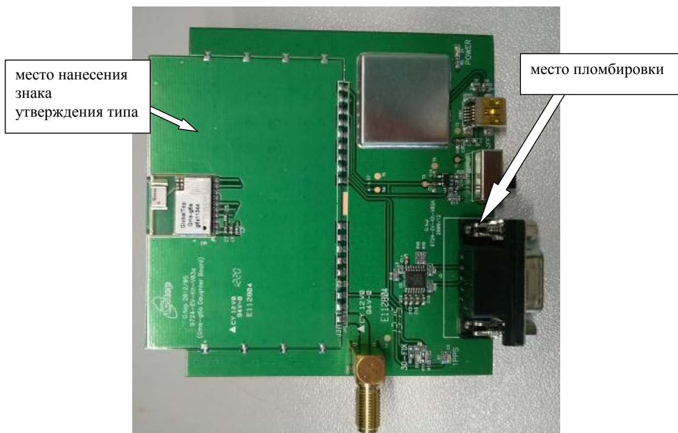
Рисунок 2 - Внешний вид аппаратуры Gms-gba
