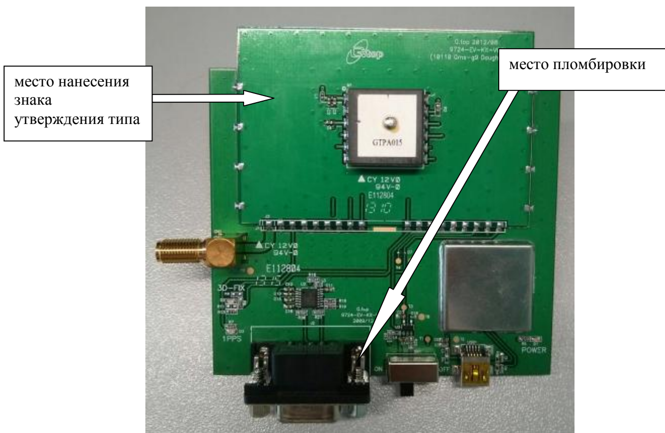
Рисунок 3 - Внешний вид аппаратуры Gms-g9
