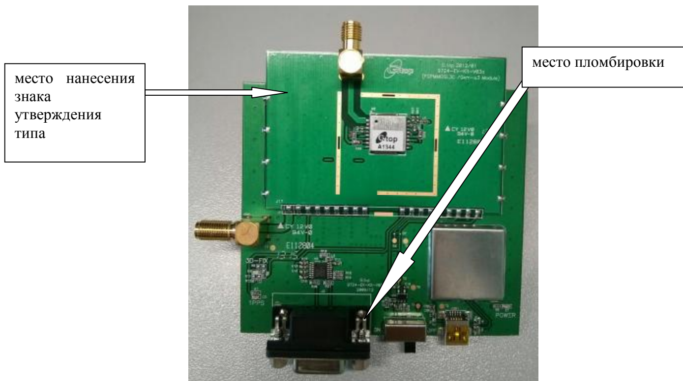
Рисунок 1 - Внешний вид аппаратуры Gmm-g3
