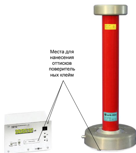
Рисунок 4 - Внешний вид киловольтметра СКВ-100-СТ
