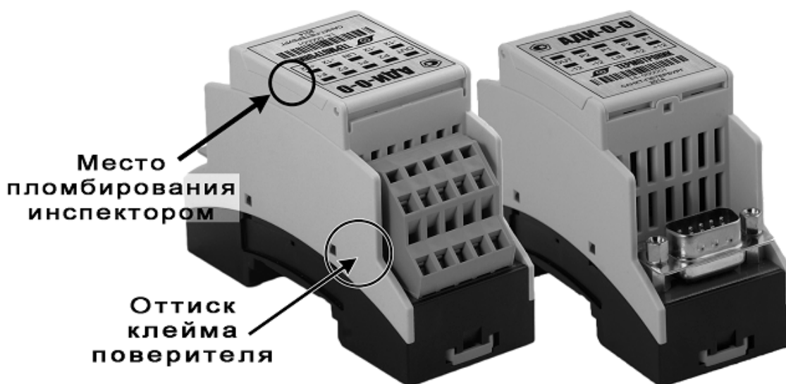
Рисунок 1 - Внешний вид АДИ и места его пломбирования
