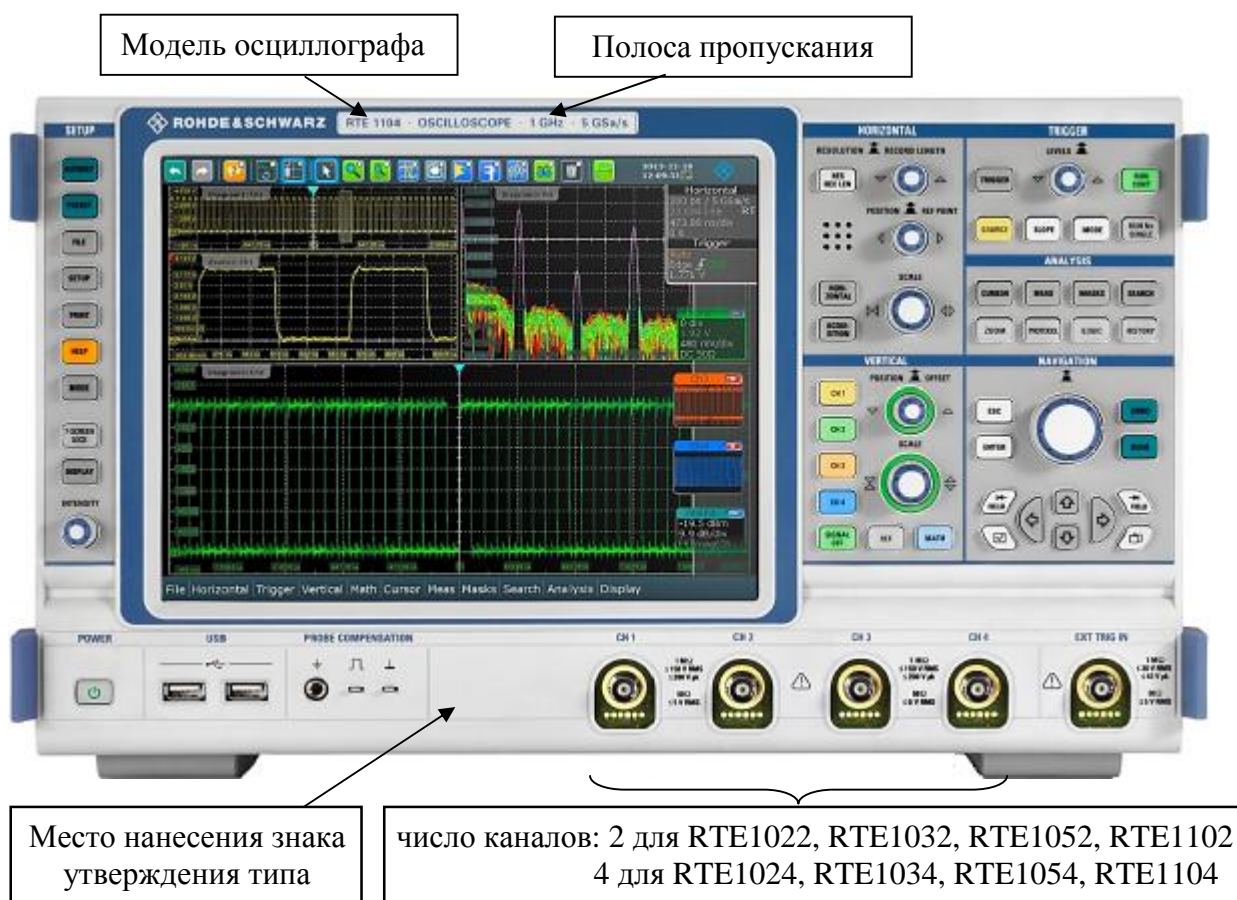
Рисунок 1 - Общий вид средства измерений
