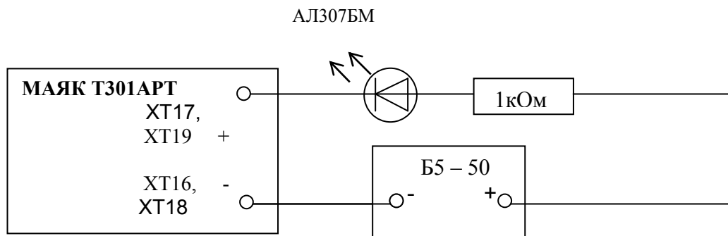
Рисунок 1 – Схема подключения светодиодного индикатора к импульсным выходам счетчика
