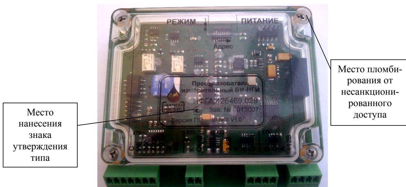
Рисунок 1 - Внешний вид преобразователя и схема пломбировки от несанкционированного доступа
