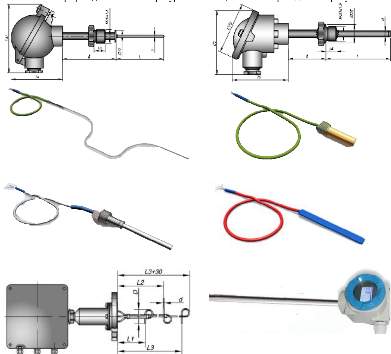
Рисунок 1 – Датчики температуры ТСПТ Ех, ТСМТ Ех
