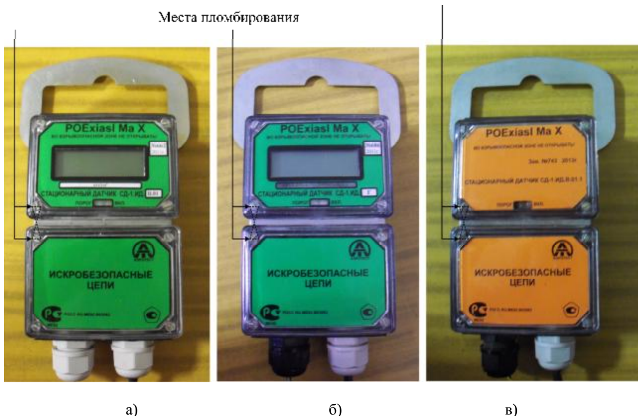
Рисунок 1. Внешний вид датчиков давления и места пломбирования корпусов. а) датчик модификации СД-1.ИД.Г, б) датчик модификации СД-1.ИД.В с жидкокристаллическим индикатором, в) и датчик модификации СД-1.ИД.В без жидкокристаллического индикатора
