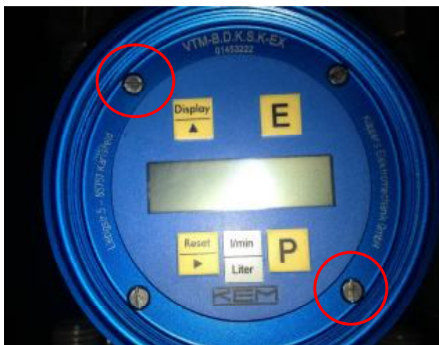
Рисунок 2 - Вычислитель расхода VTM-B.D.K.S/K-Ex
