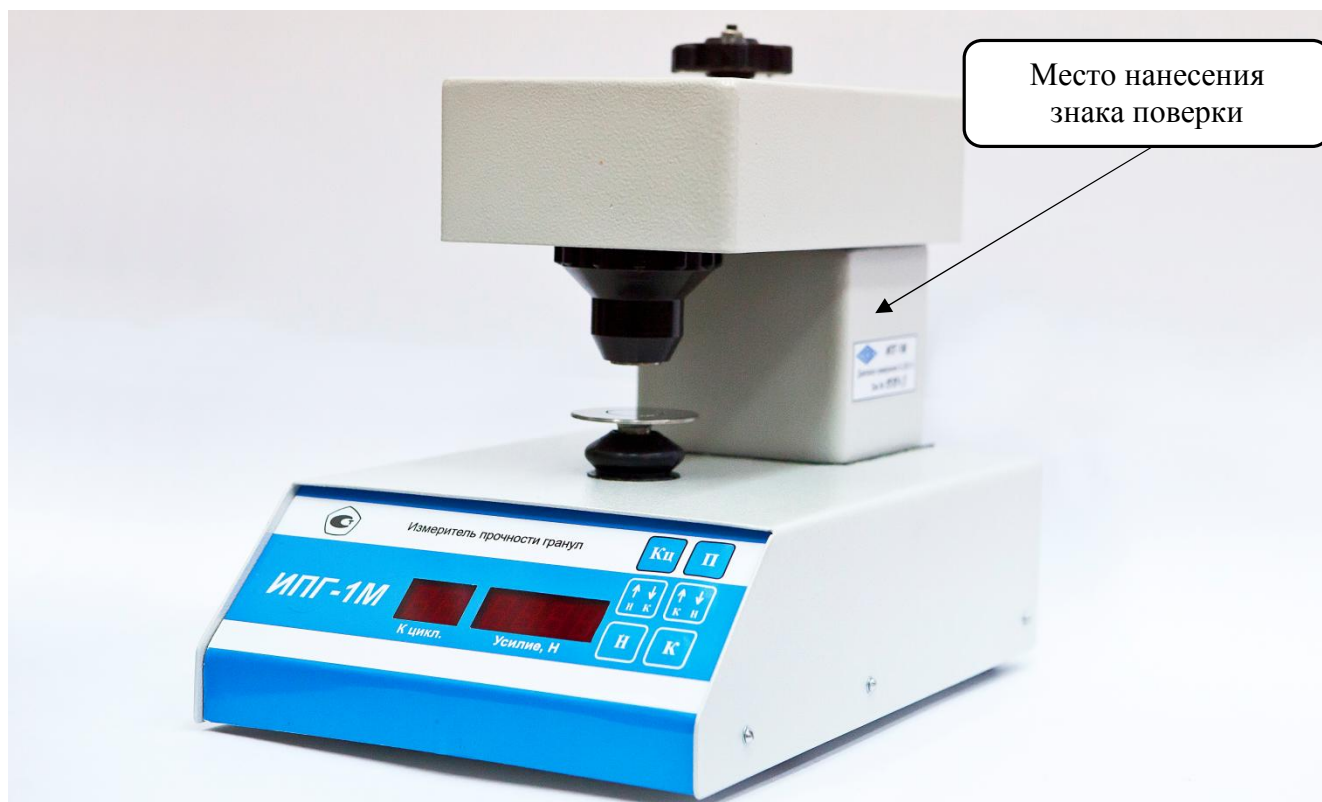
Рисунок 1 – Общий вид приборов
