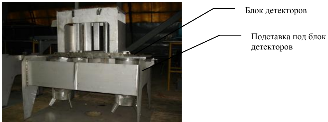
Рисунок 1 - Внешний вид блока детекторов
