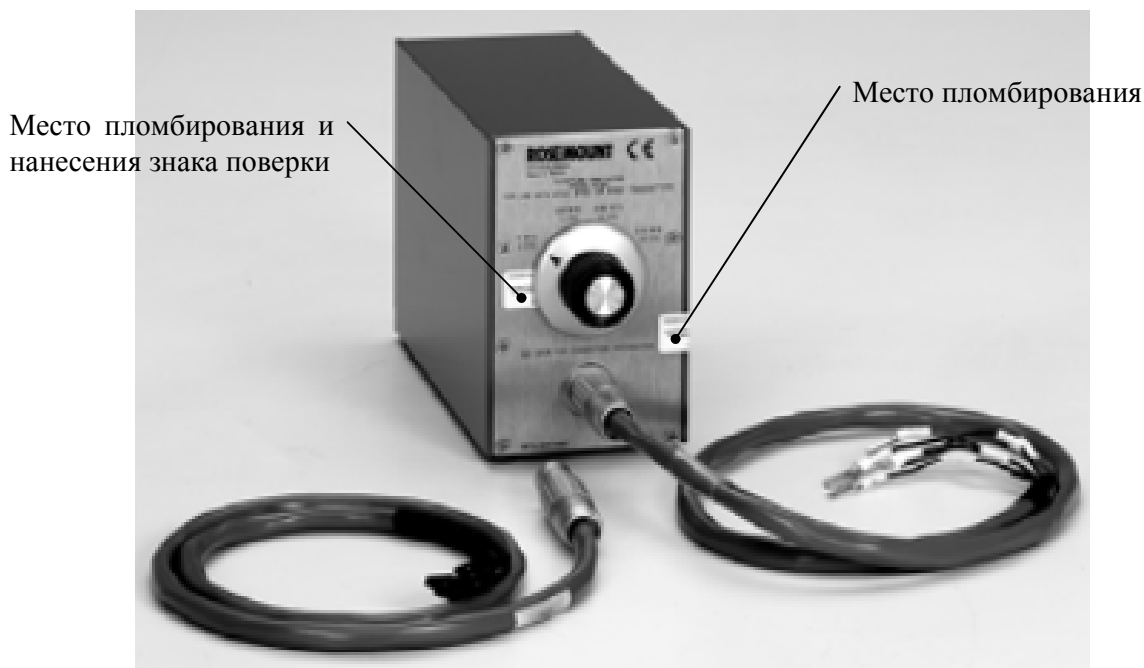
Рисунок 1 – Внешний вид имитатора 8714
