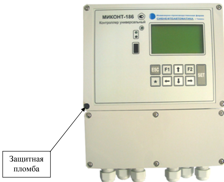
Рисунок 1– Схема пломбировки контроллера МИКОНТ-186 от несанкционированного доступа.
