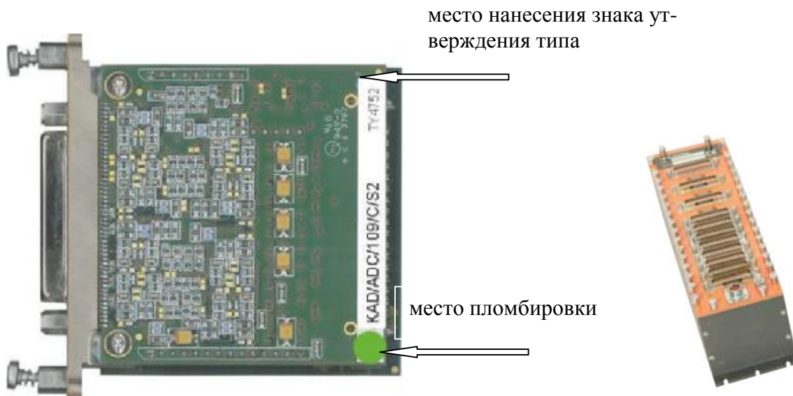
Рисунок 1 - Внешний вид модуля KAD/ADC/109/C/S2, модуля KAD/ADC/109/C/S2, модуля KAD/ADC/109/C/S1 и модуля KAM/ADC/109/C/S1, установленного в блок базовый KAM/CHS/13U
