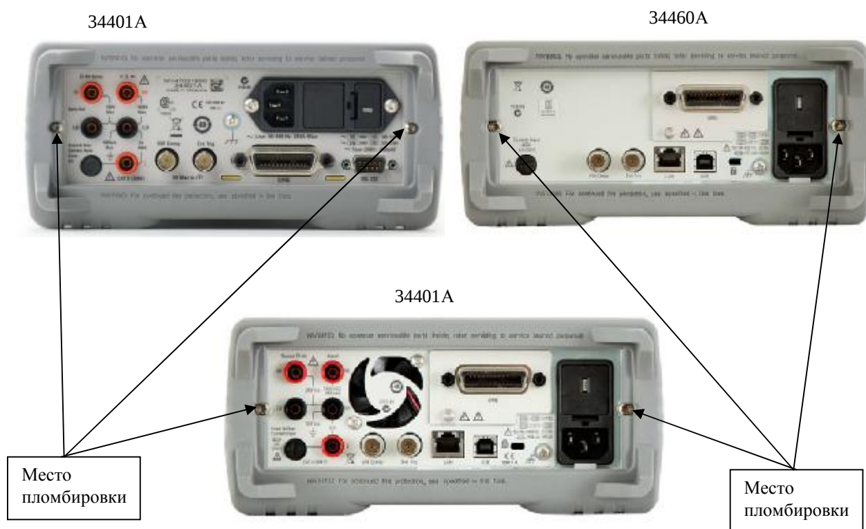
Рисунок 2 - Задние панели мультиметров
