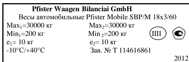
Рисунок 4 Маркировка на весоизмерительных устройствах
