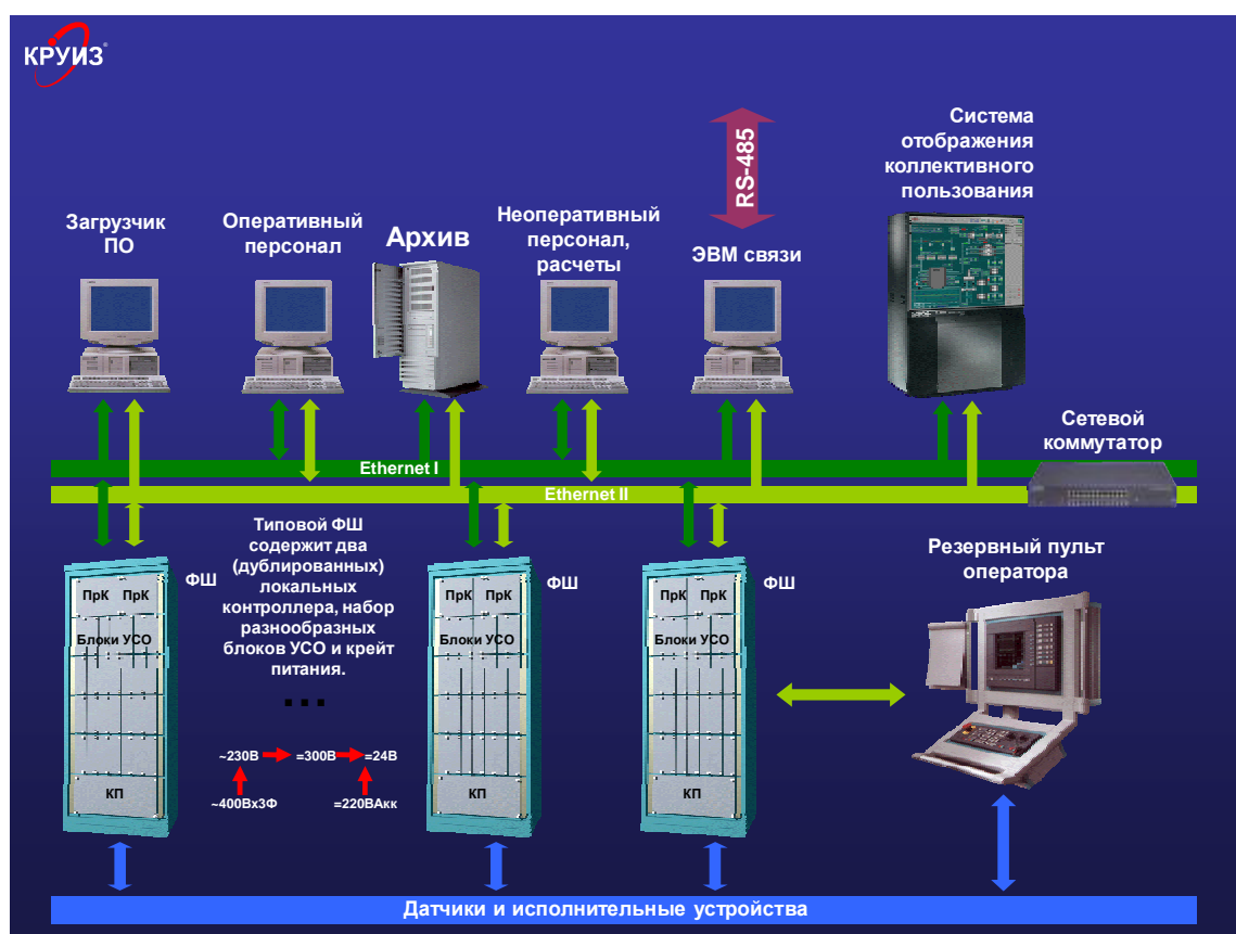
Рисунок 1 – Структурная схема
